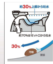
従来型ゼット口付便器
